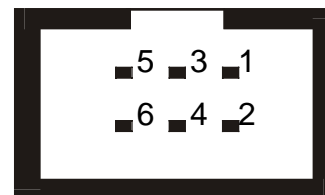
FIGURA 8: CONNETTORE ISP DELL'MP AVR-51+
