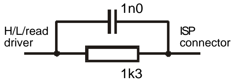
FIGURA 7: DRIVER ISP DELL'MP AVR-51+
