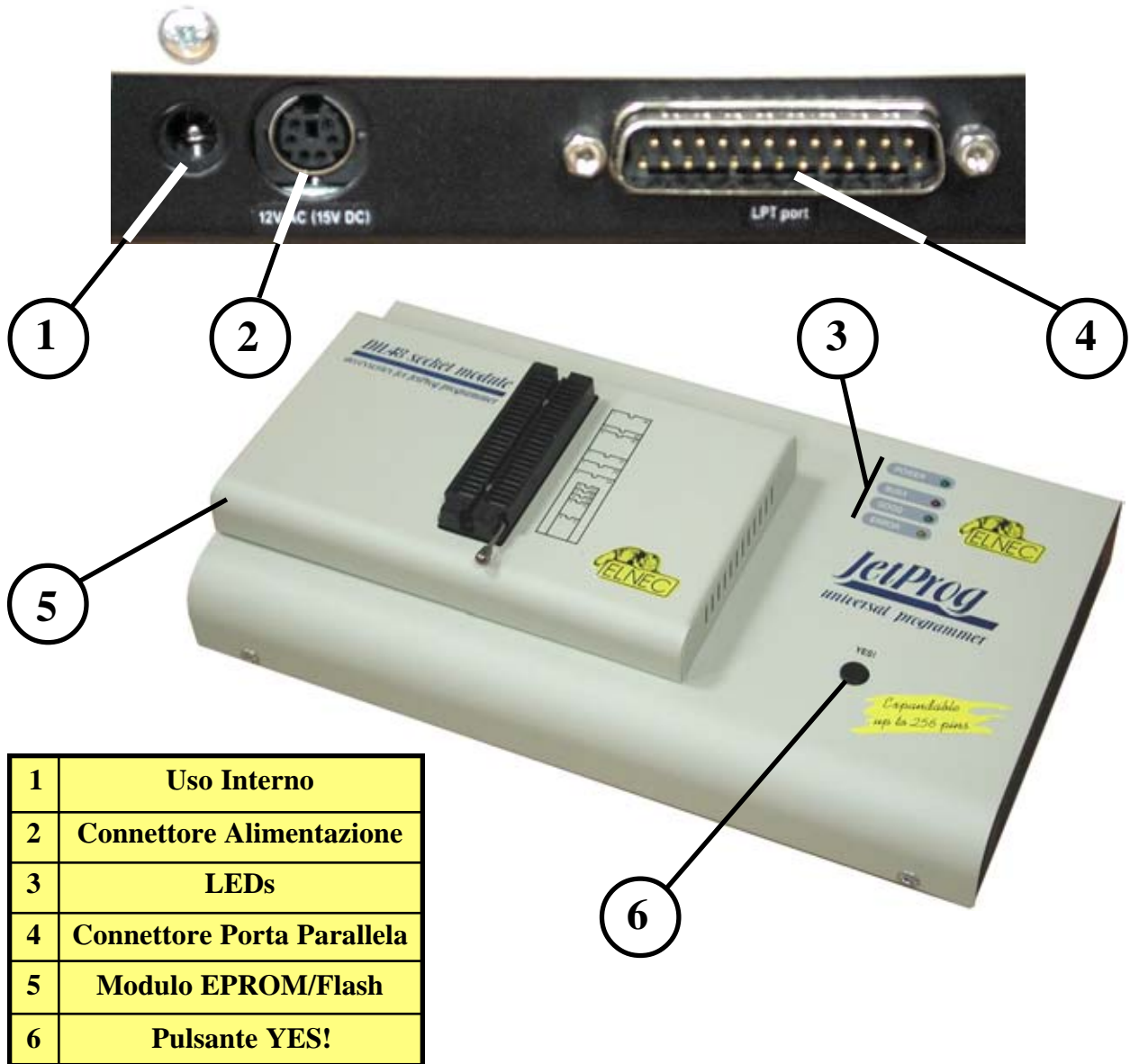
FIGURA 7: PIANTA DEGLI ELEMENTI
