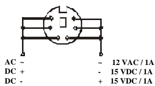
FIGURA 9: CONNETTORE DI ALIMENTAZIONE
