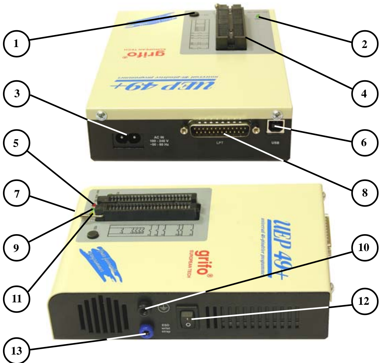
FIGURA 4: POSIZIONE LEDs, CONNETTORI, PULSANTE, ECC.
