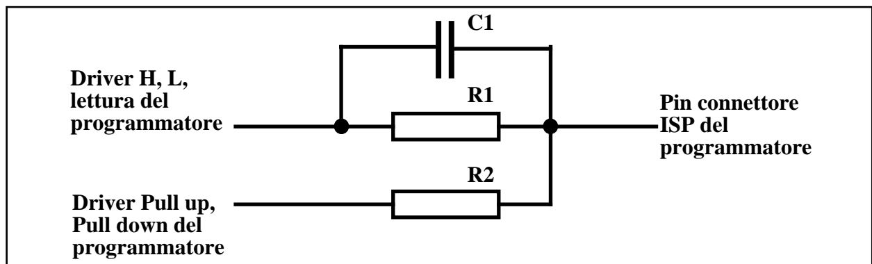
FIGURA 15: COLLEGAMENTO SEGNALI ISP SU PROGRAMMATORE
