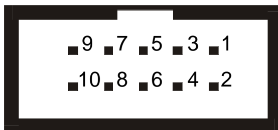
FIGURA 13: CONNETTORE ISP
