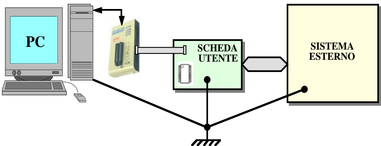
FIGURA 12: COLLEGAMENTO PER PROGRAMMAZIONE ISP
