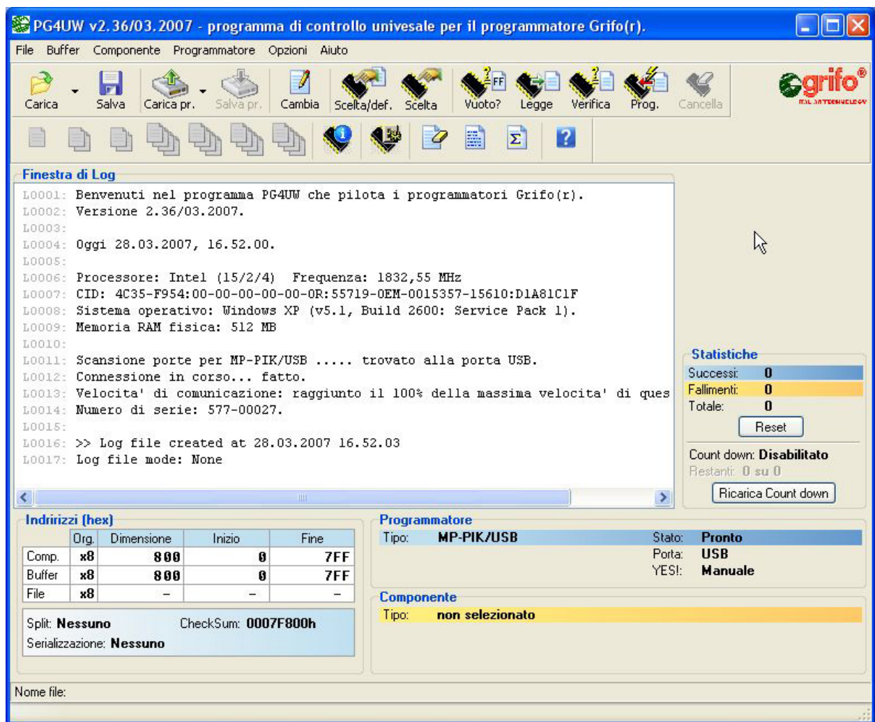
FIGURA 16: FINESTRA PRINCIPALE PG4UW
