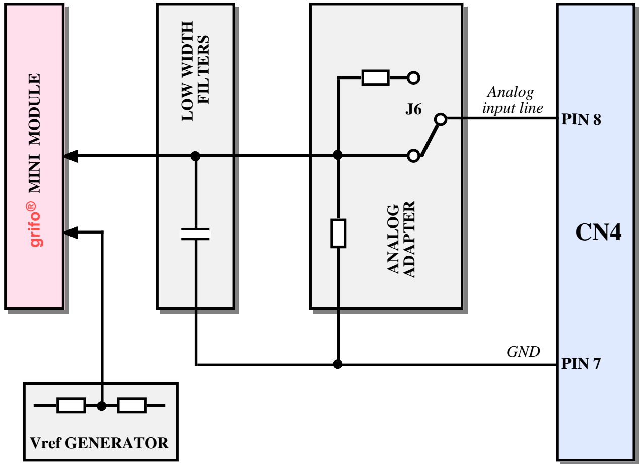
FIGURA 26: SCHEMA COLLEGAMENTO INGRESSO ANALOGICO A/D
