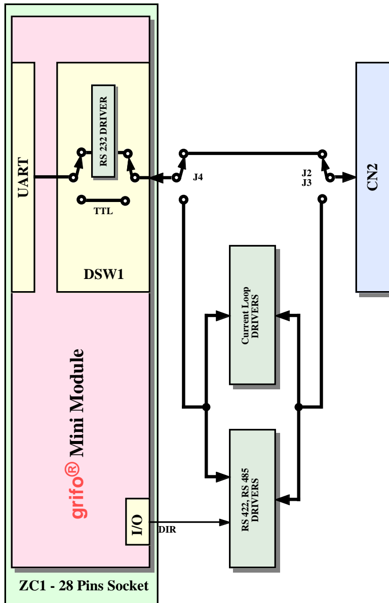
FIGURA 10: SCHEMA DI COMUNICAZIONE SERIALE
