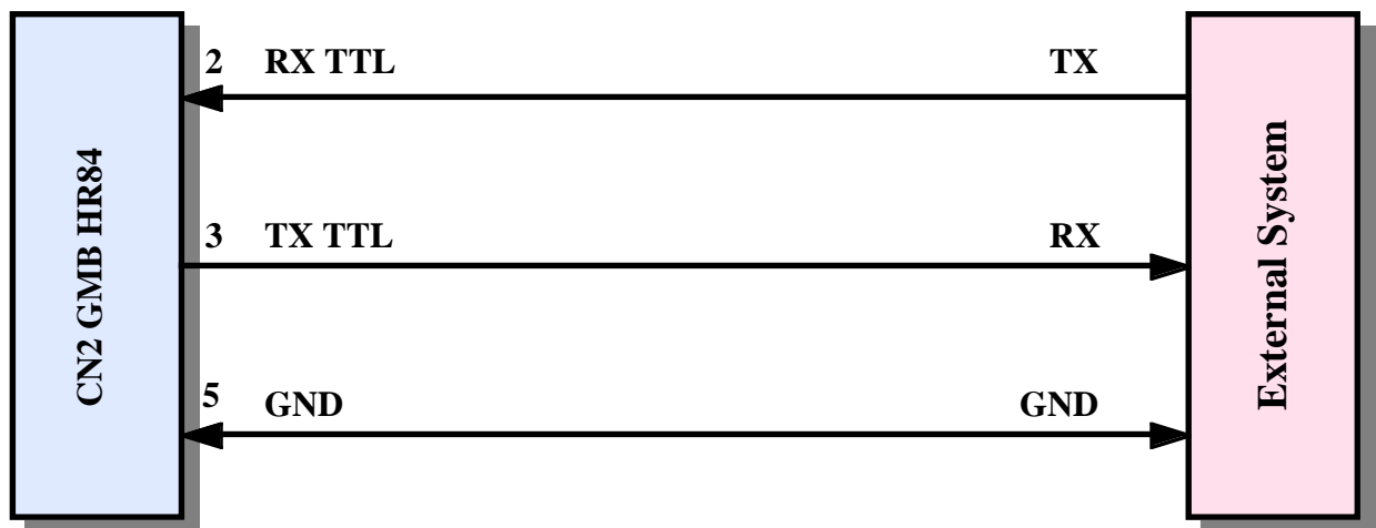
FIGURA 27: ESEMPIO DI COLLEGAMENTO LINEA SERIALE TTL
