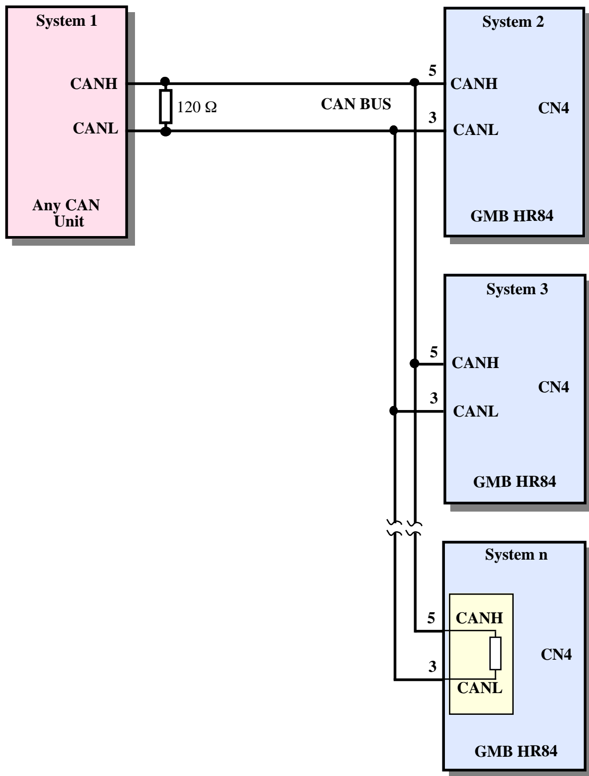
FIGURA 28: ESEMPIO COLLEGAMENTO RETE CAN
