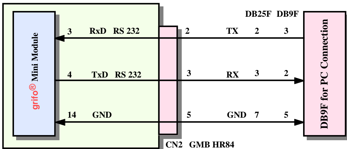
FIGURA 11: ESEMPIO COLLEGAMENTO PUNTO PUNTO IN RS 232 E TTL
