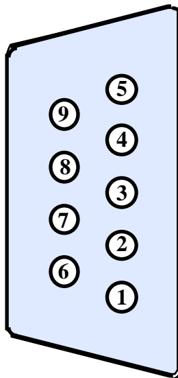
FIGURA 9: CN2 - CONNETTORE PER LINEA SERIALE
