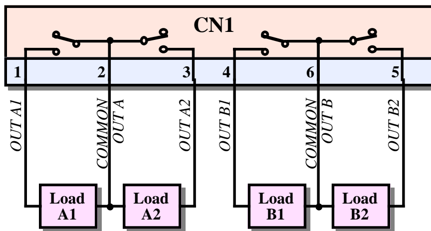
FIGURA 24: SCHEMA DI COLLEGAMENTO DELLE USCITE A RELÉ' A E B
