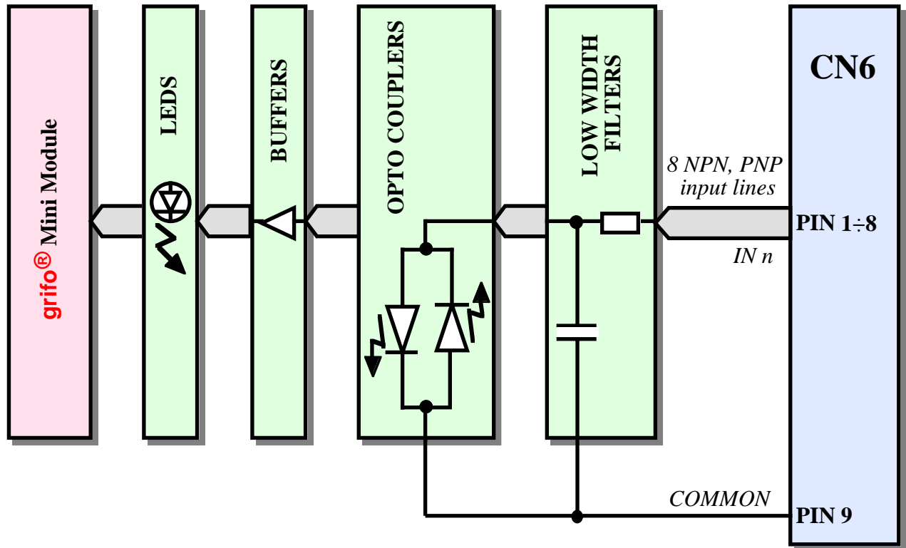
FIGURA 20: SCHEMA DEGLI INGRESSI OPTOISOLATI
