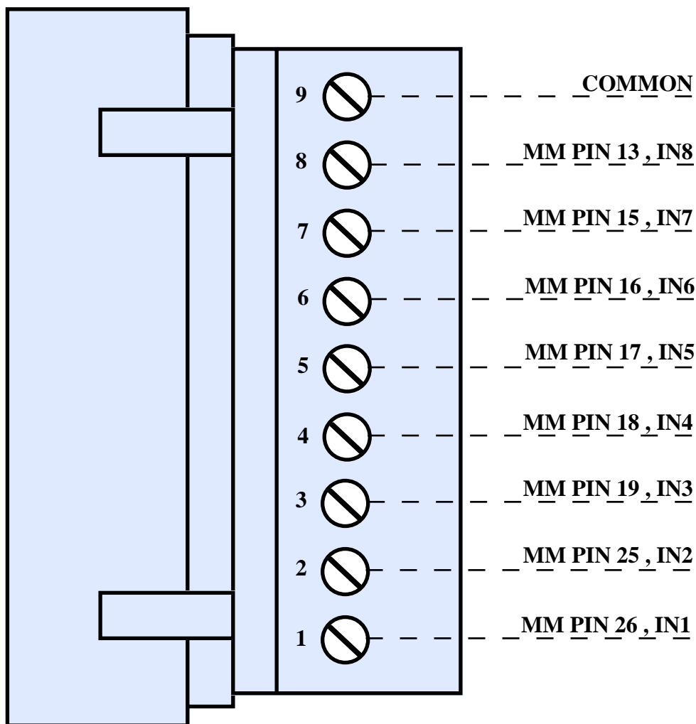
FIGURA 19: CN6 - CONNETTORE PER INGRESSI OPTOISOLATI
