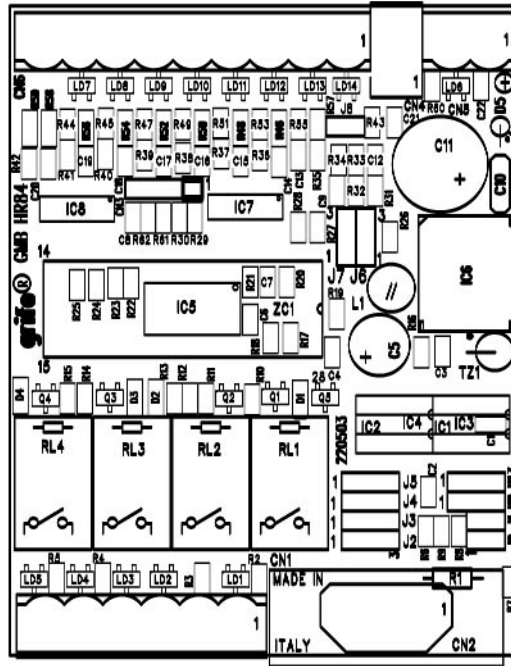
FIGURA 30: PIANTA COMPONENTI (LATO COMPONENTI)
