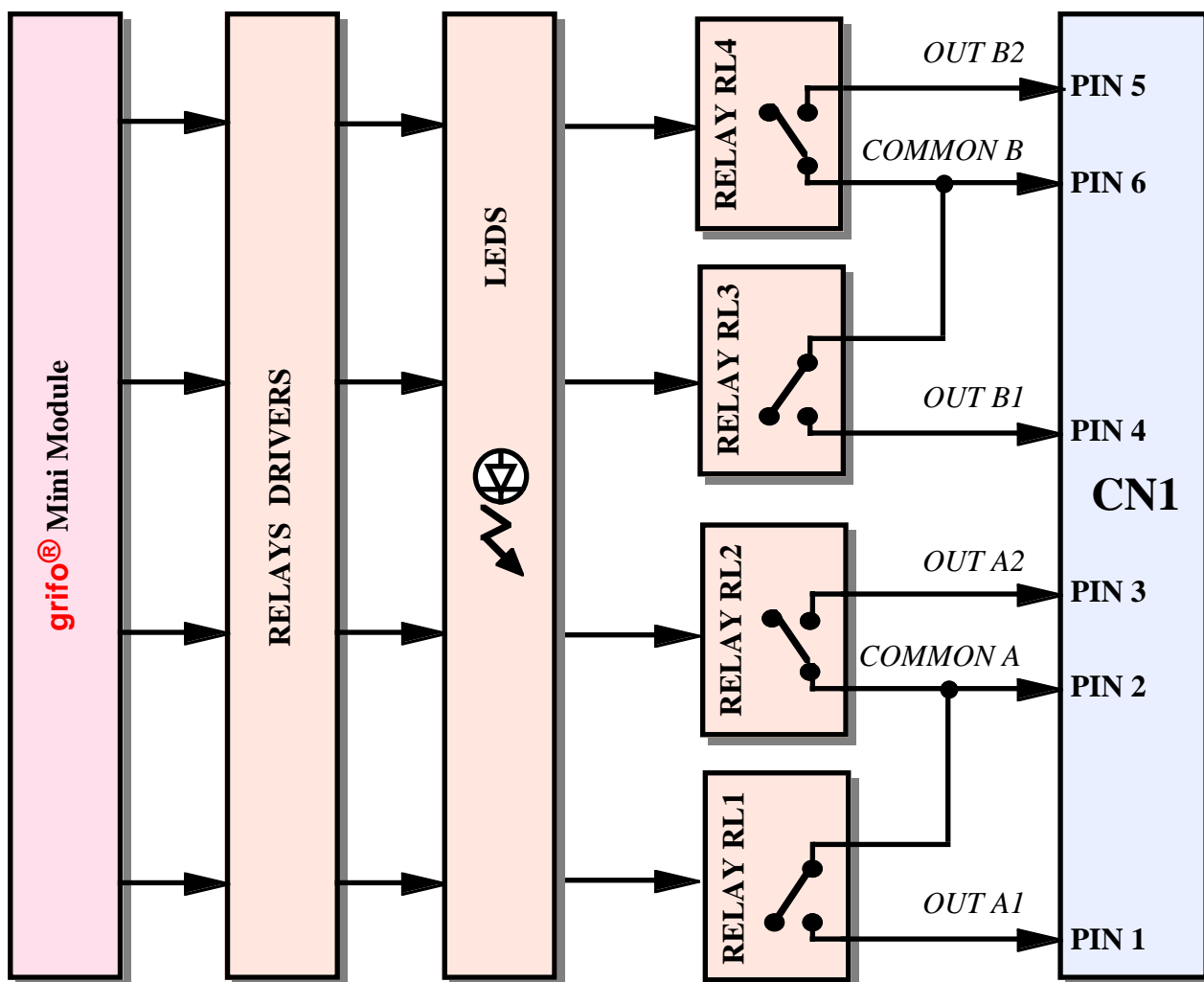
FIGURA 23: SCHEMA DELLE USCITE A RELÉ A E B
