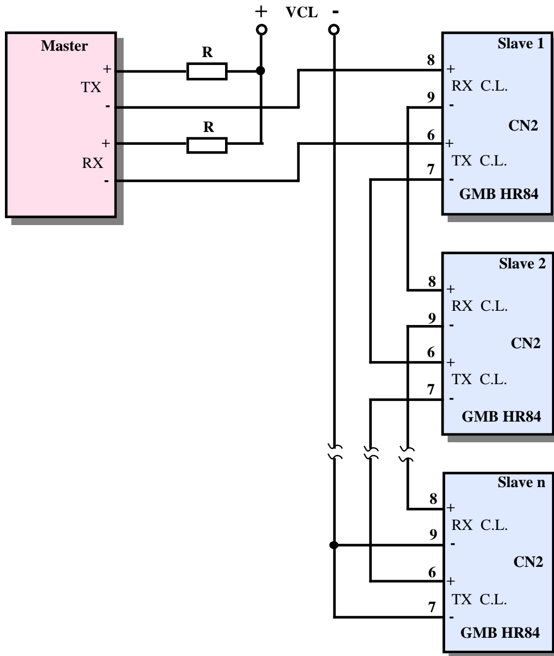
FIGURA 18: ESEMPIO DI COLLEGAMENTO IN RETE IN CURRENT LOOP
