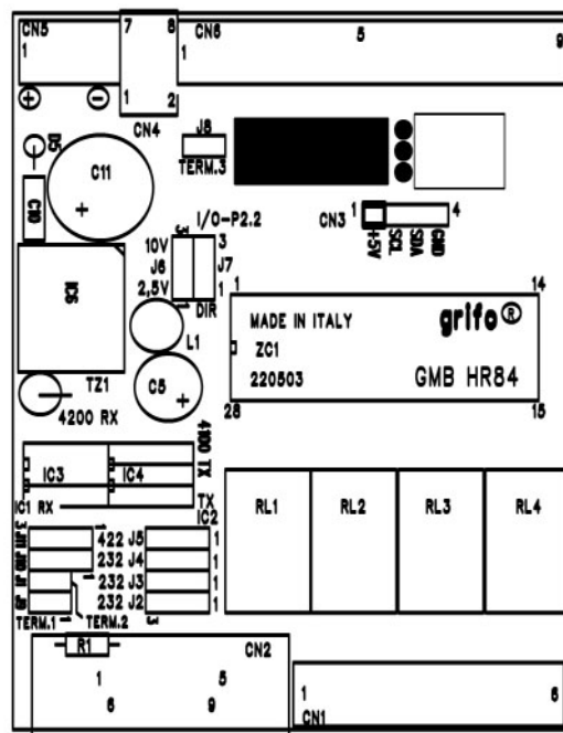
FIGURA 31: PIANTA COMPONENTI (LATO STAGNATURE)
