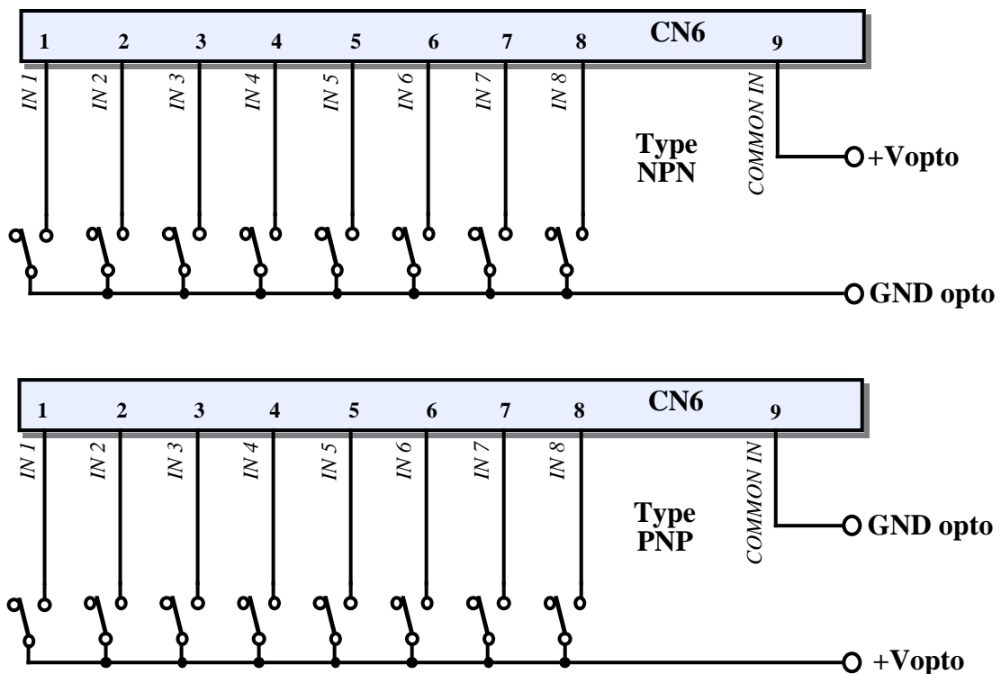
FIGURA 21: SCHEMA DI COLLEGAMENTO DEGLI INGRESSI OPTOISOLATI
