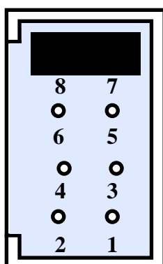
FIGURA 38: ATTIVAZIONE PROGRAMMAZIONE ISP DA CN4
