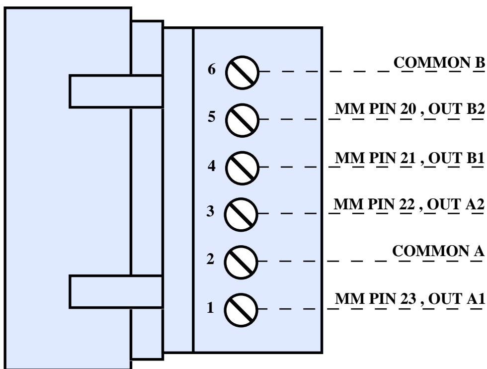
FIGURA 22: CN1 - CONNETTORE PER USCITE A RELÈ GRUPPI A E B
